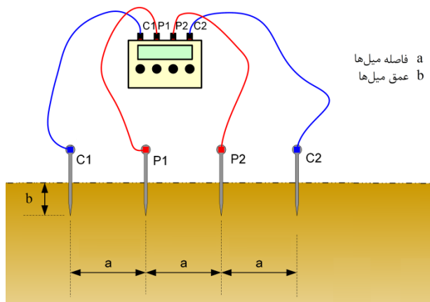
شکل (۱۵): اندازه‌گیری مقاومت ویژه خاک به روش ورنر
