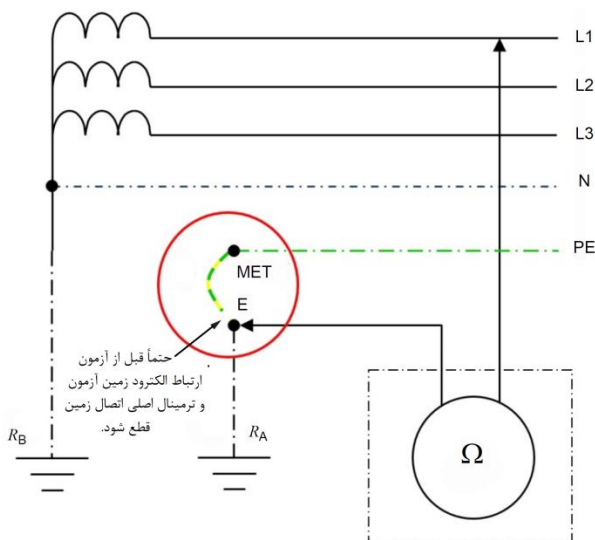
شکل (۱۳): اندازه‌گیری مقاومت الکتروود زمین با استفاده از دستگاه آزمون امیدانس حلقه
