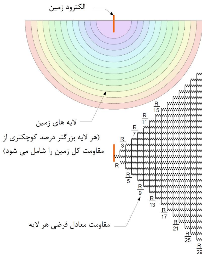
شکل (۱۷): مدار معادل پیوسته‌های هم‌پتانسیل طرف یک الکترو
