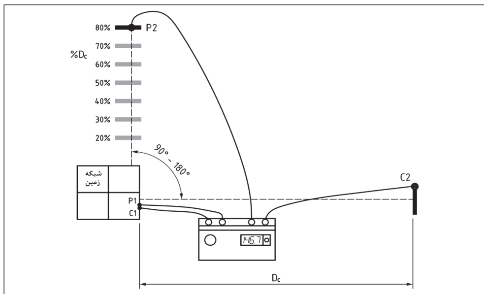
شکل (۷): آزمون 90^\circ/180^\circ
